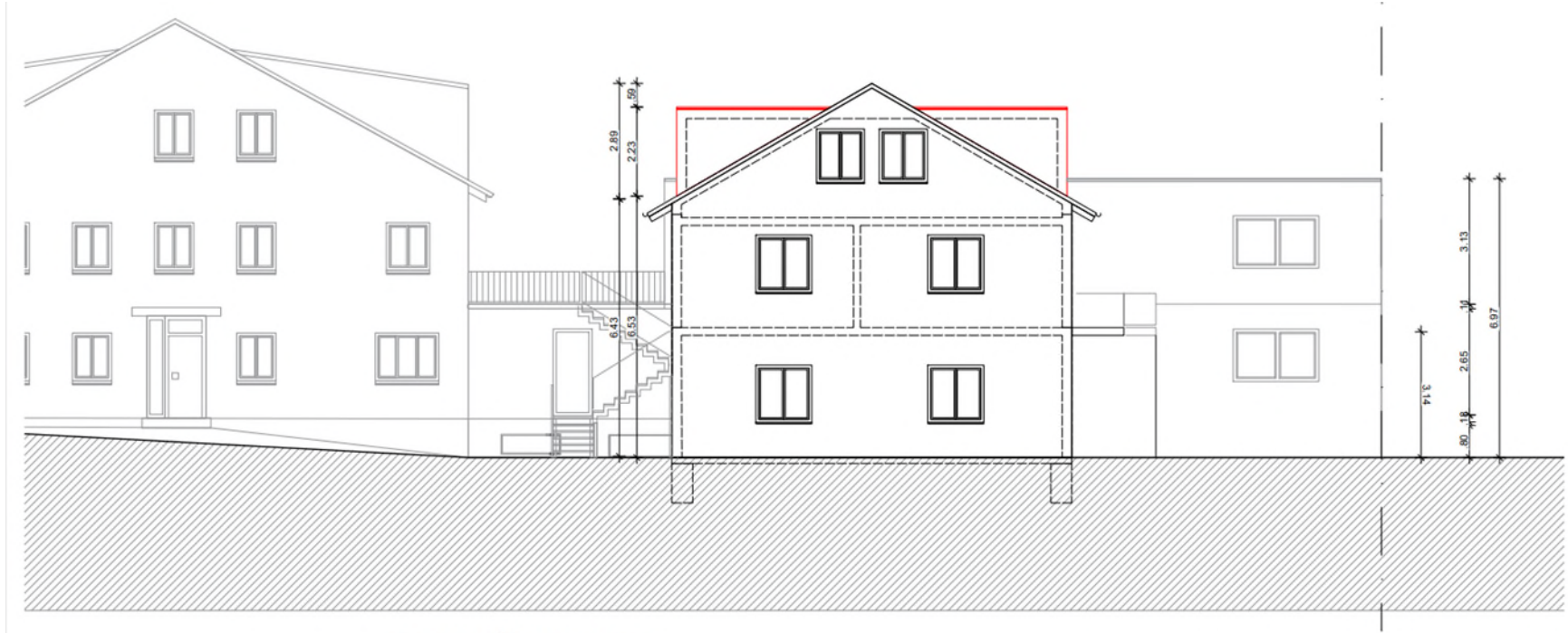
Ansicht SÜD Wohnhaus
