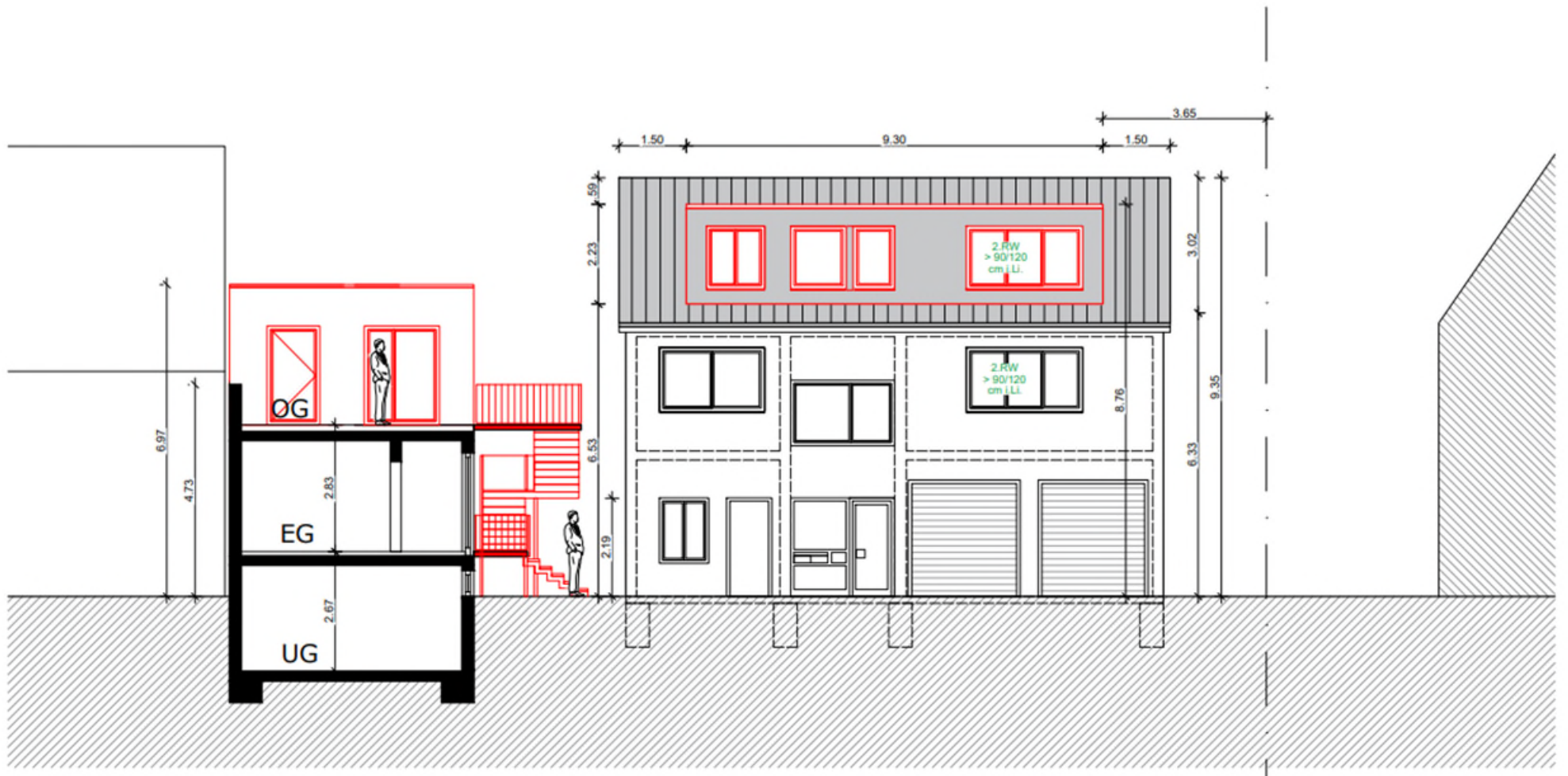
Schnitt B - B, Ansicht WEST Wohnhaus
